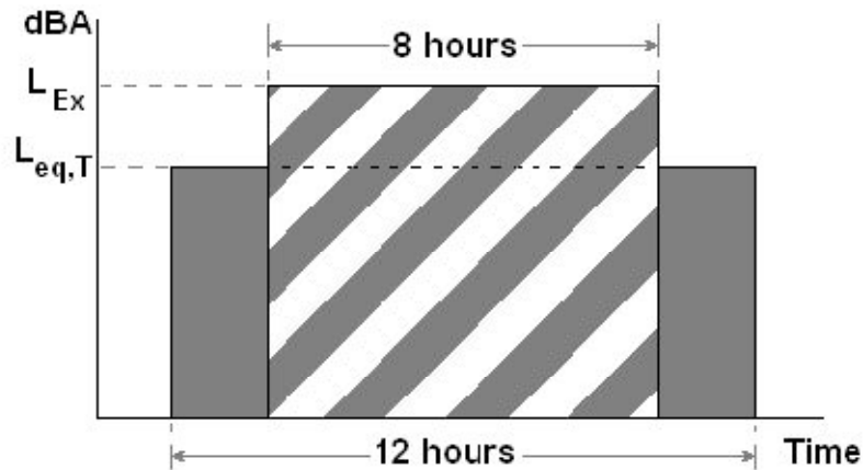
شکل : تبدیل شیفت 12 ساعته به LEX شیفت 8 ساعته استاندارد مقدار LEX طبق فرمول زیر برابر است با :
